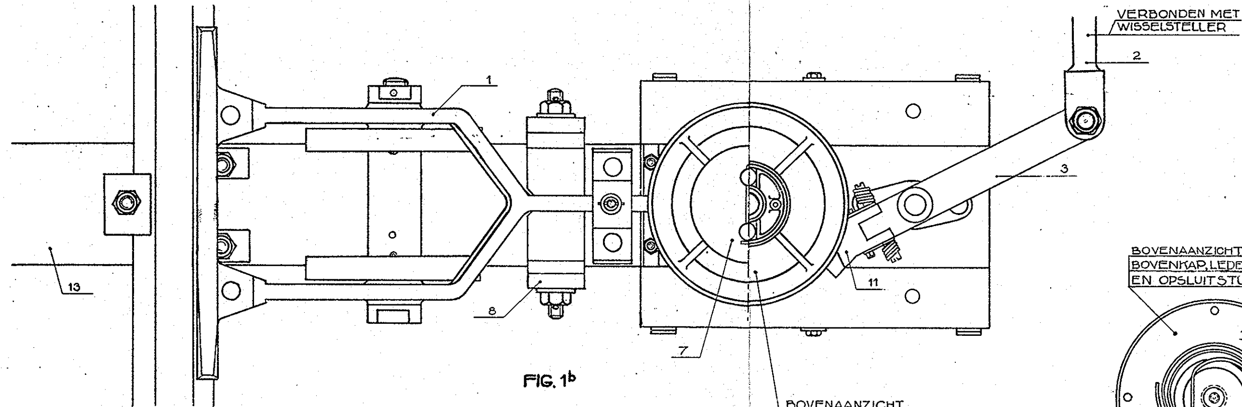
BOVENAANZICHT ZONDER DEKSEL 7
