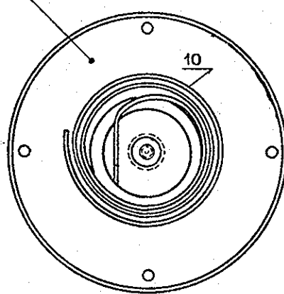
BOVENAANZICHT ZONDER BOVENKAP, LEDEREN BODEM EN OPSLUITSTUK
