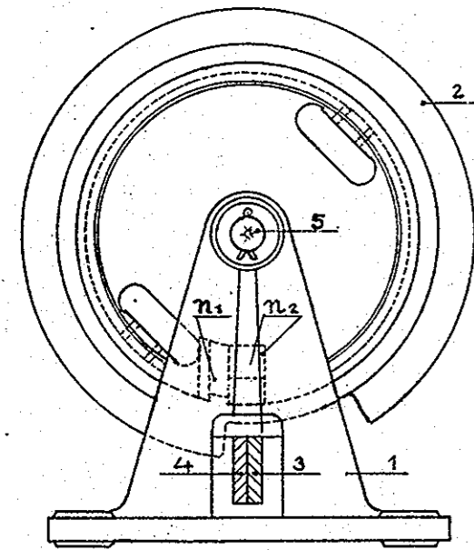
FIG. 1 c (DOORSNEDE A-B)
