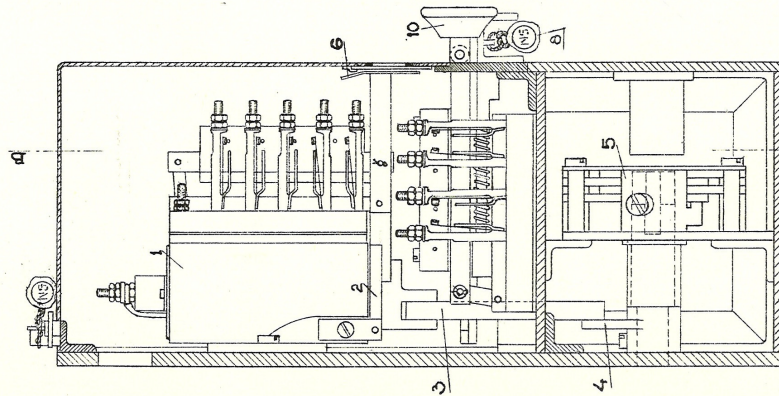
DOORSNEDE C-D FIG. 1a
