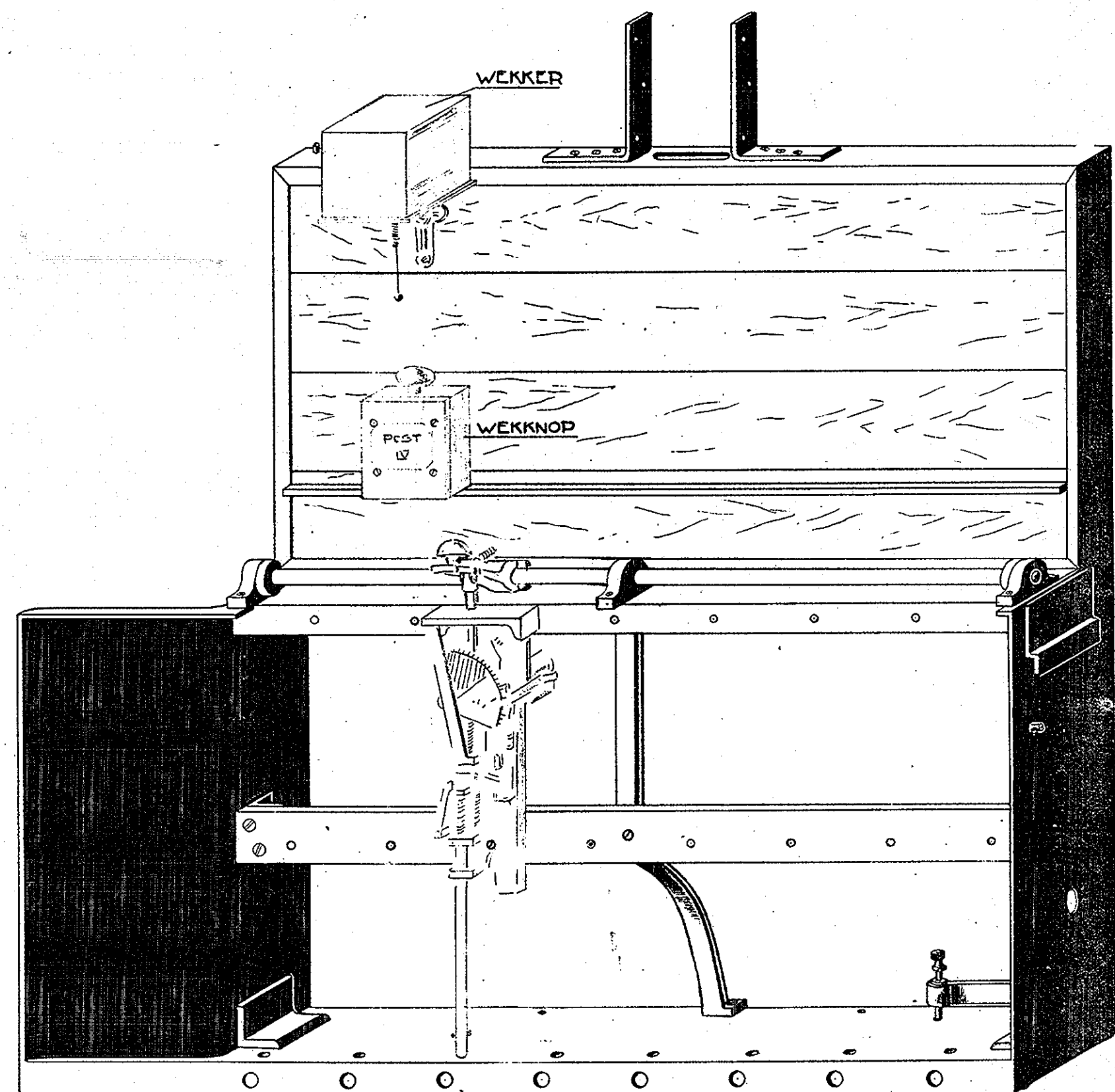
FIG.1 BLOKKAST GEZIEN VAN VOORZUDE (VOOR-EN ACHTERWAND AFGENOMEN)
