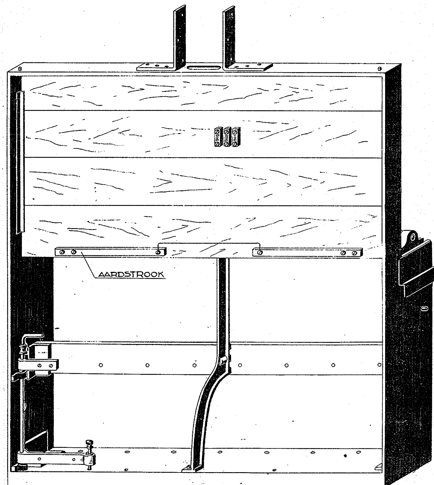
FIG.2 BLOKKAST GEZIEN VAN ACHTERZUDE (VOOR-EN ACHTERWAND AFGENOMEN)
